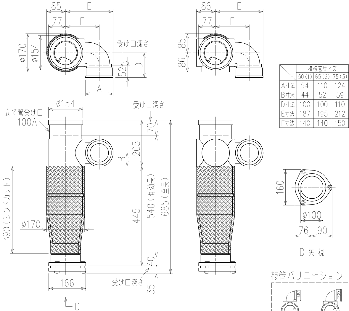
両受けスタイル (W) + シンドカット ※ 対応スラブ厚 180~380
