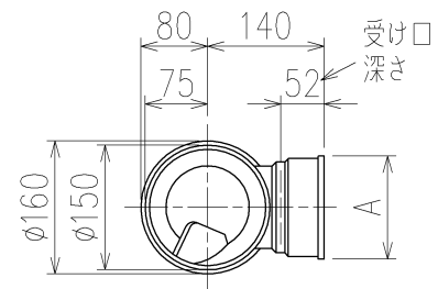
C-C断面矢視
