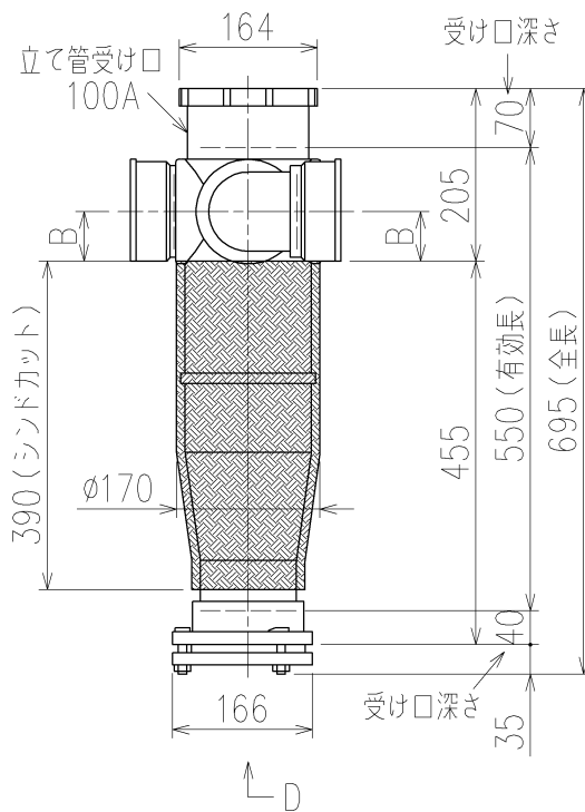
両受けスタイル (W) + シンドカット ※ 対応スラブ厚 180~380
