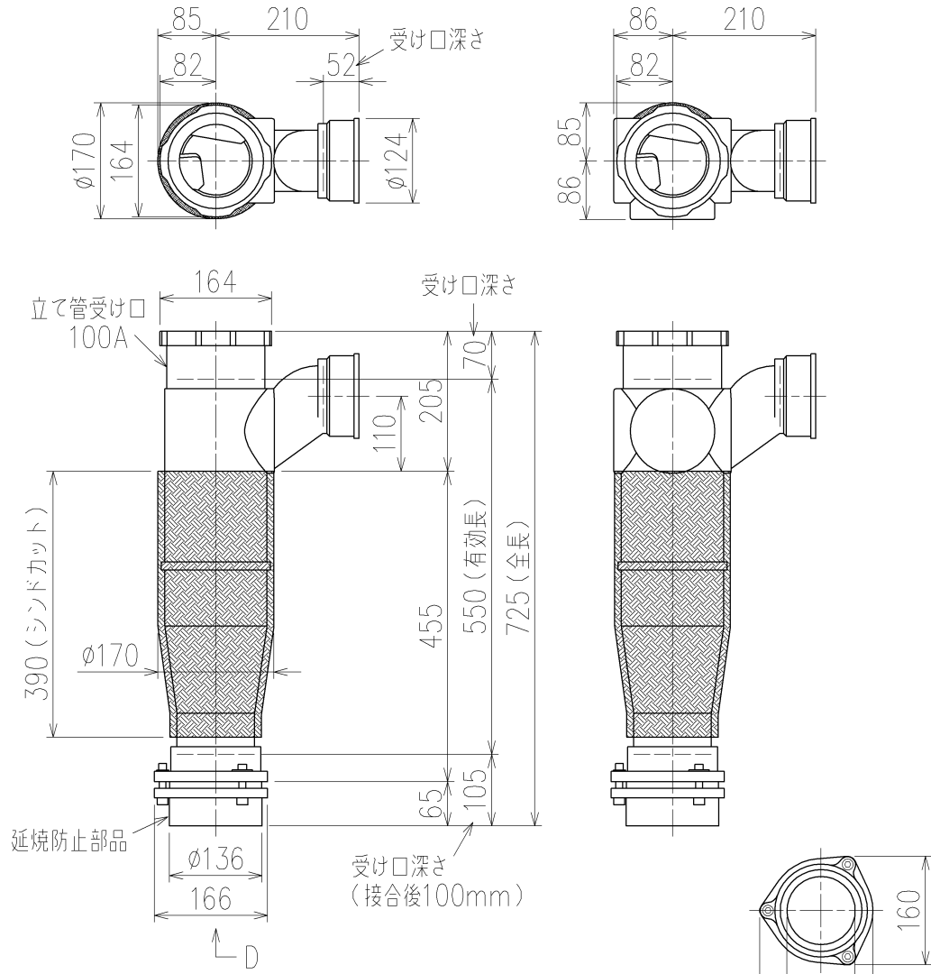
カンペイ君 (WKP) + シンドカット ※ 対応スラブ厚 150~380
