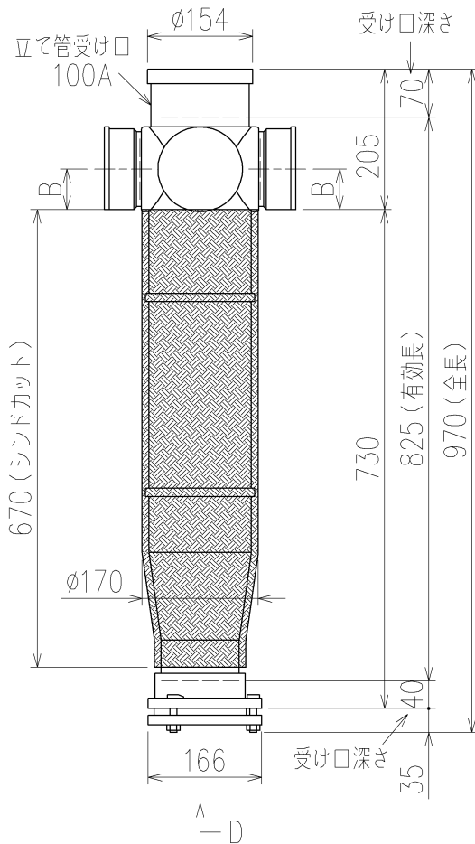
両受けスタイル (W) + シンドカット ※ 対応スラブ厚 180~660
