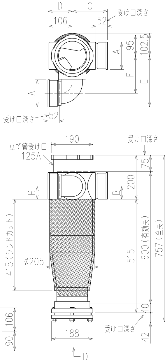
両受けスタイル(W) + シンドカット ※ 対応スラブ厚 180~405
