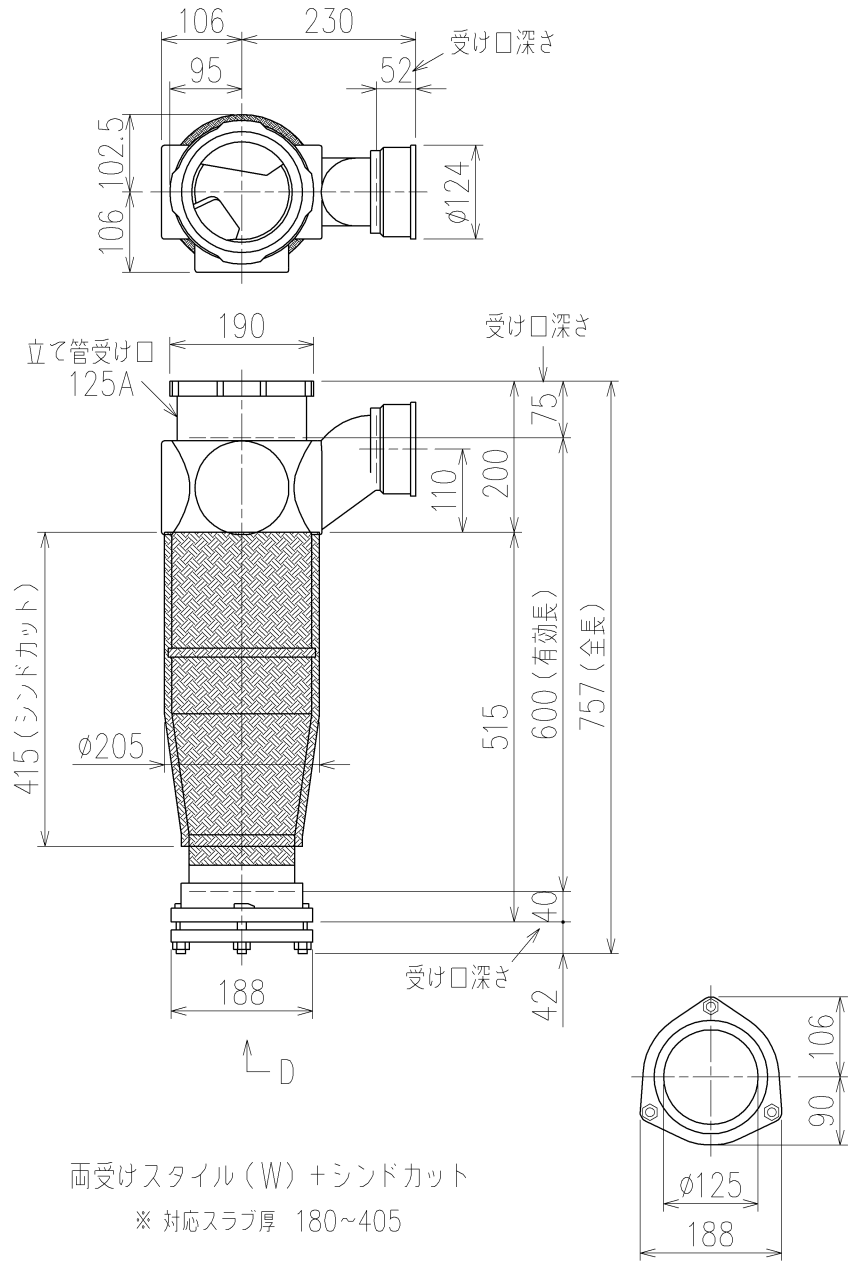
D 矢視
