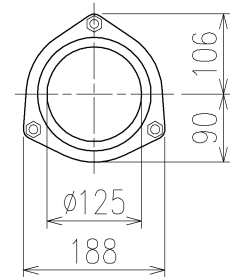
D 矢視
