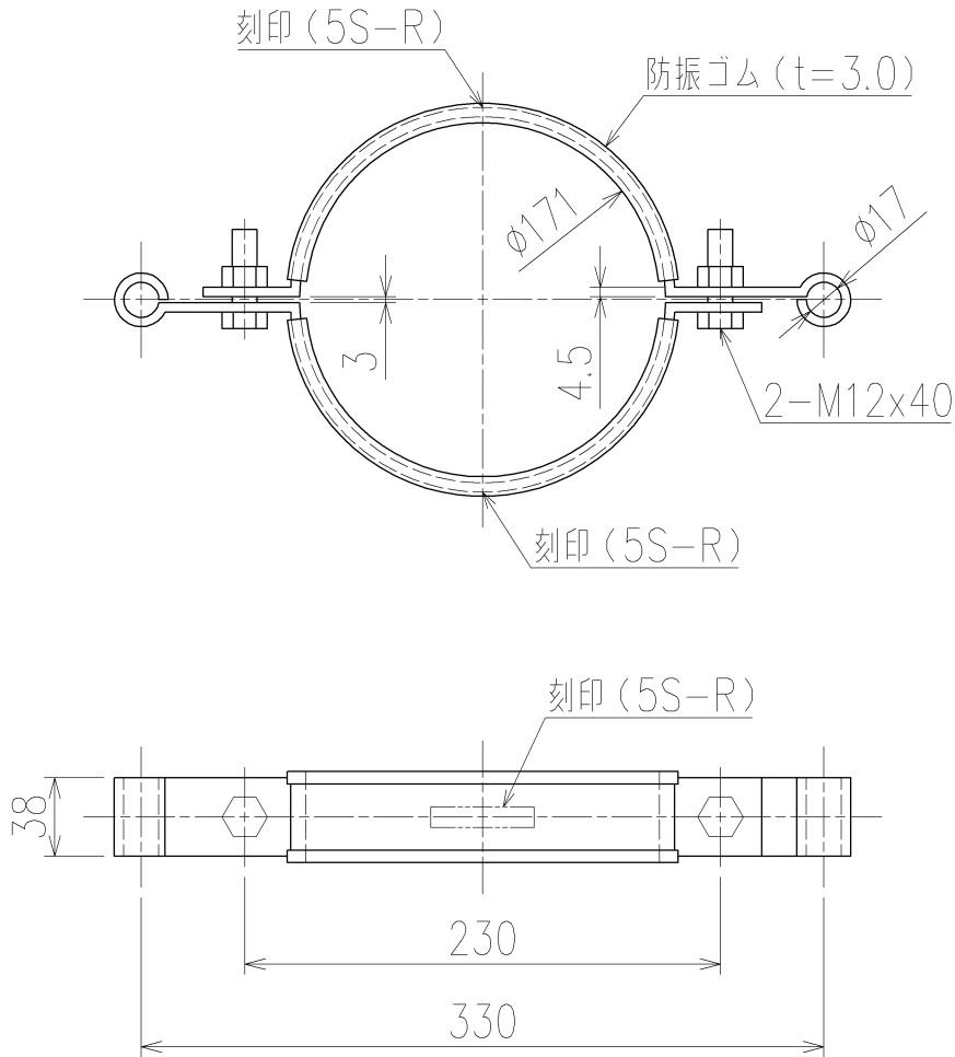
5HF/コンパクト5Lバンド用、ゴム付 (鋼、電気めっき)
