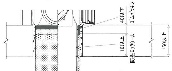
図3 防振ロックウール及びゴムパッキンの幅
