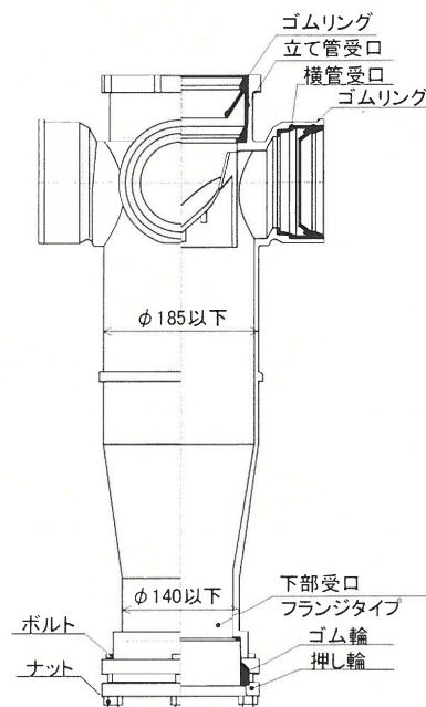
図4 排水集合管の構造 (代表例)
