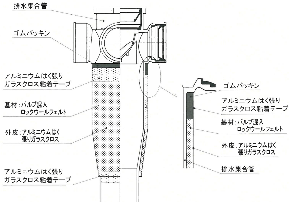
図1 防振ロックウール付排水集合管（代表例）
