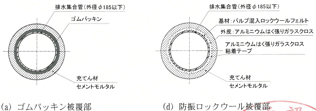
図2 区画貫通部の断面
