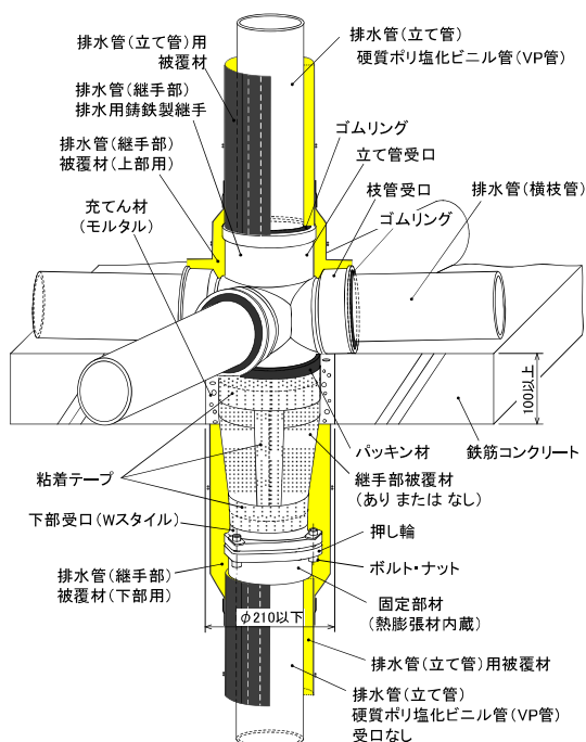
(1) 排水管(立て管)が硬質ポリ塩化ビニル管 (VP 管) 受口なしの場合
