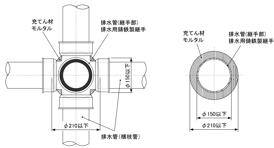
上面図
