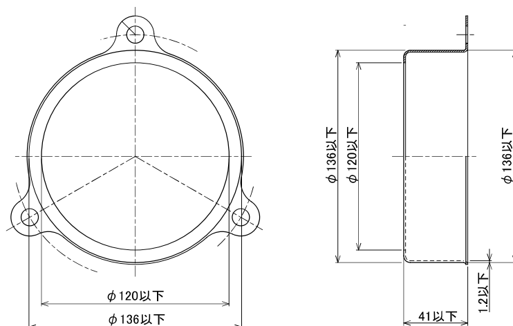
上面図
