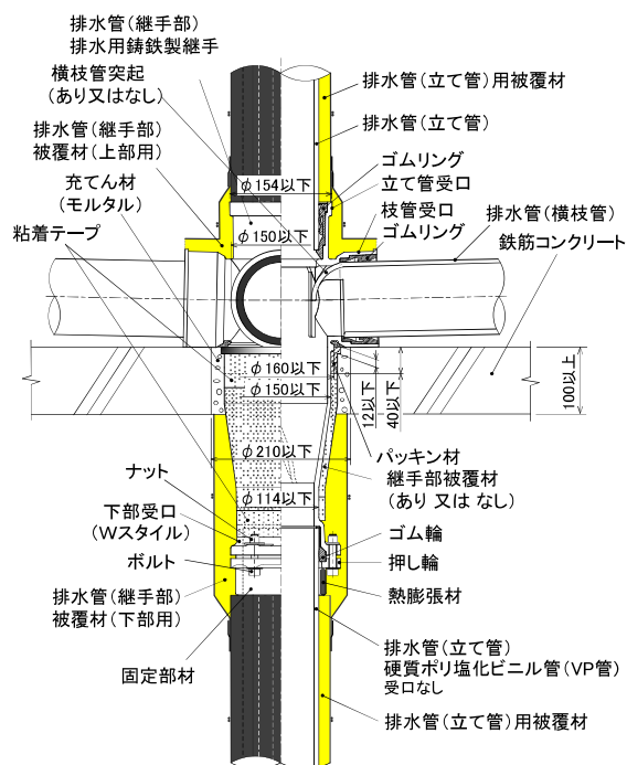
(1) 排水管(立て管)が硬質ポリ塩化ビニル管(VP管)受口なしの場合
