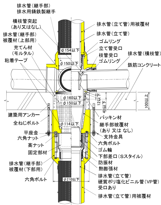
(1) 支持金具がAタイプの場合
