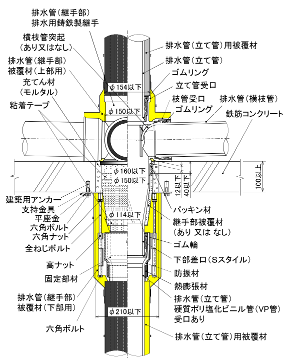
(2) 支持金具がBタイプの場合
