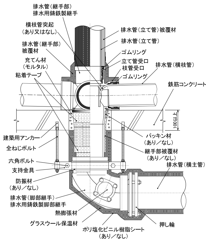
(1) 立て管側受口：差込み形受口の場合
