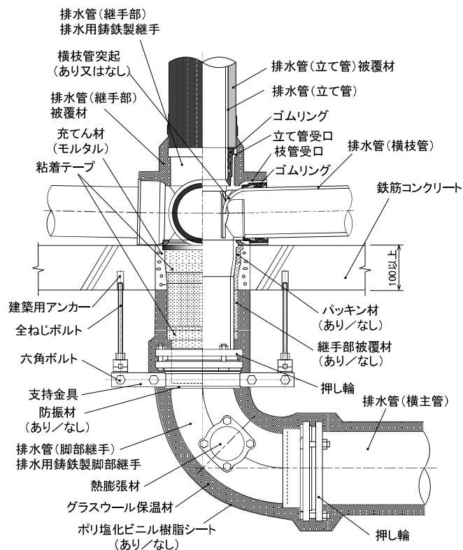
(2) 立て管側受口：メカニカル形受口の場合
