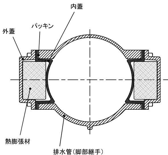
A-A断面
