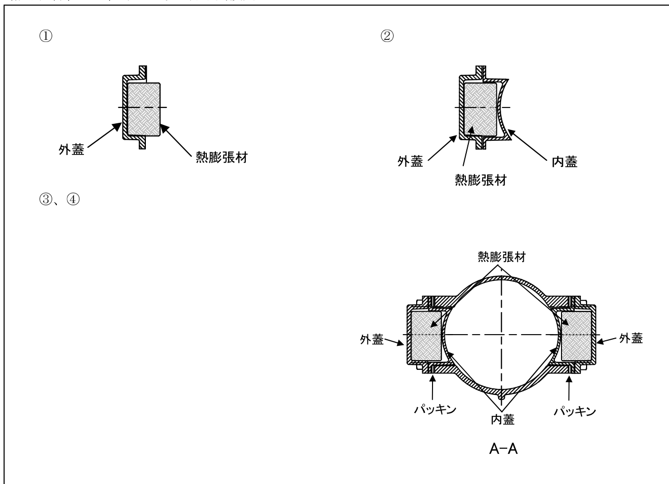
熱膨張材、内蓋、外蓋の取り付け要領図
