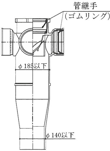
管継手(ストレートタイプ)の詳細図(代表例)
