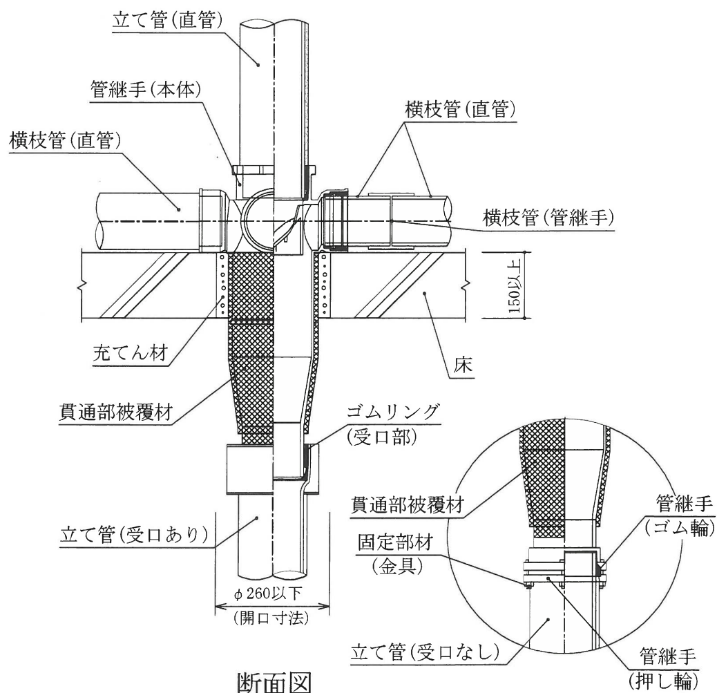
図1 構造説明図（施工図）
