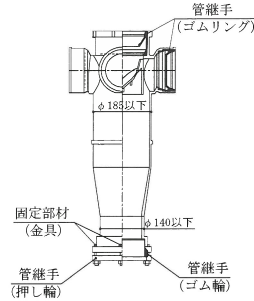
管継手(フランジタイプ)の詳細図(代表例)
