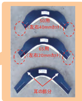
②枝部クボタイカバーを枝管受口にセットします。 50～75用はサイズにより両端を切り落として使用します。
