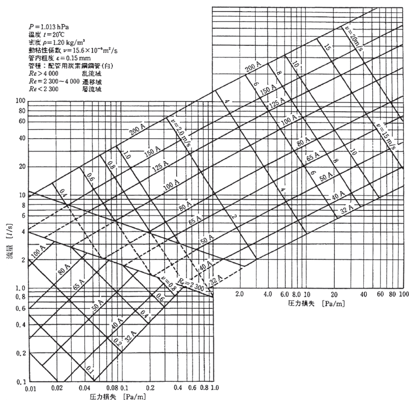
図7 通気管損失線図 (SHASE-S206)
