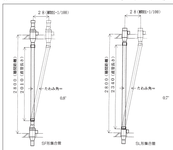
図9 集合管方式の層間変位対応性
